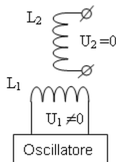
Fig.1 Queste bobine ortogonali non interagiscono.
